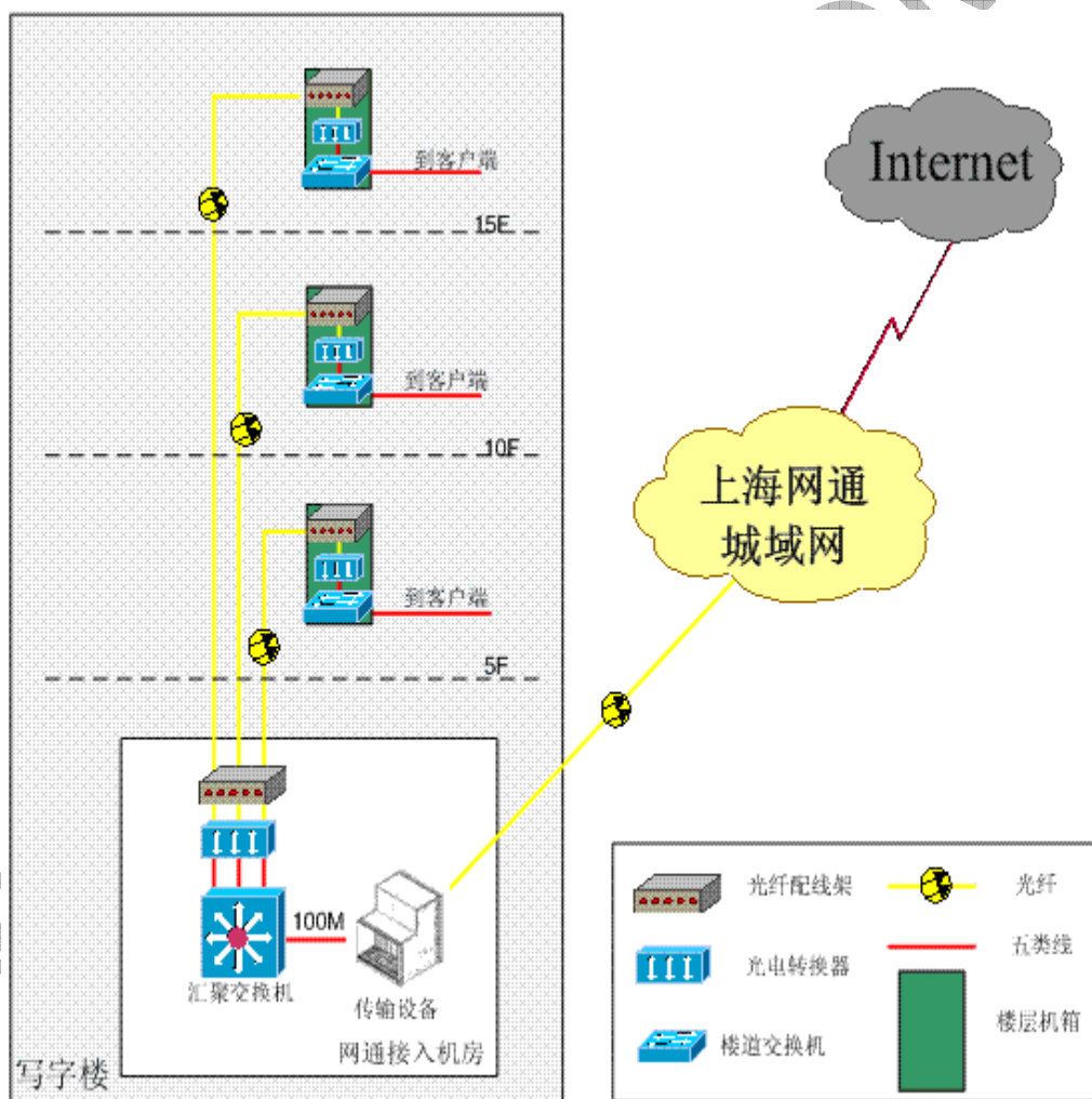
网通 DIA 接入方式示意图
